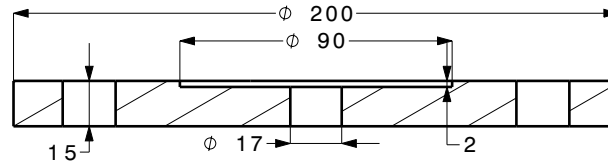
Section view Z-Z Scale: 2:5
