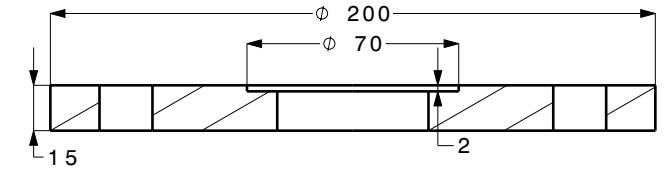
Section view AA-AA Scale: 2:5
