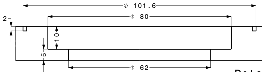
Detail R Scale: 1:1
