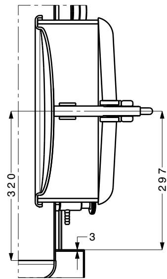
Section view M-M Scale: 1:8
