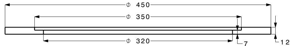
Section view U-U Scale: 1:4
