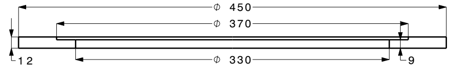
Section view S-S Scale: 1:4
